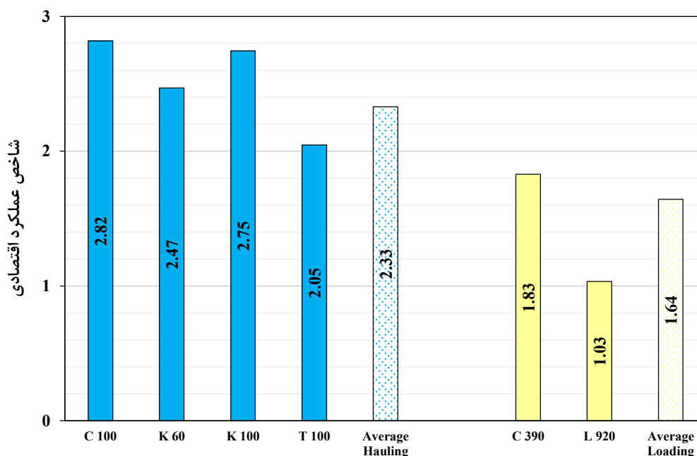
شکل ۵: شاخص عملکرد اقتصادی ماشین آلات ناوگان بارگیری و باربری
