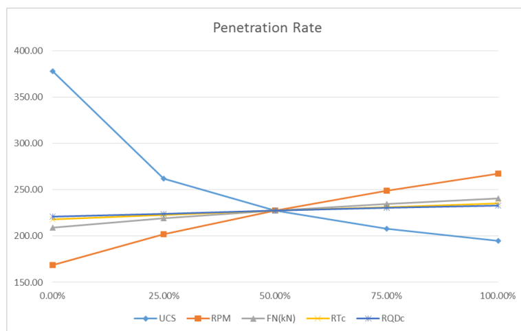
شکل ۱۲: نمودار گردباد تحلیل حساسیت مدل فرخ و همکاران
