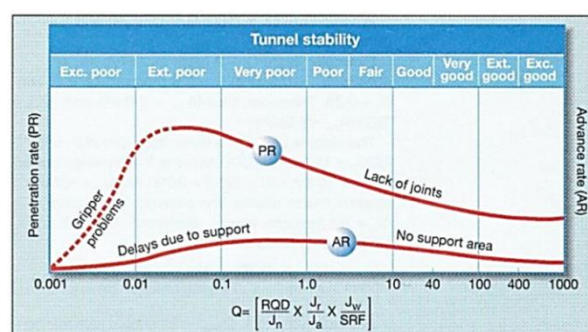
شکل ۴: رابطه بین PR و Q [۲۳]
