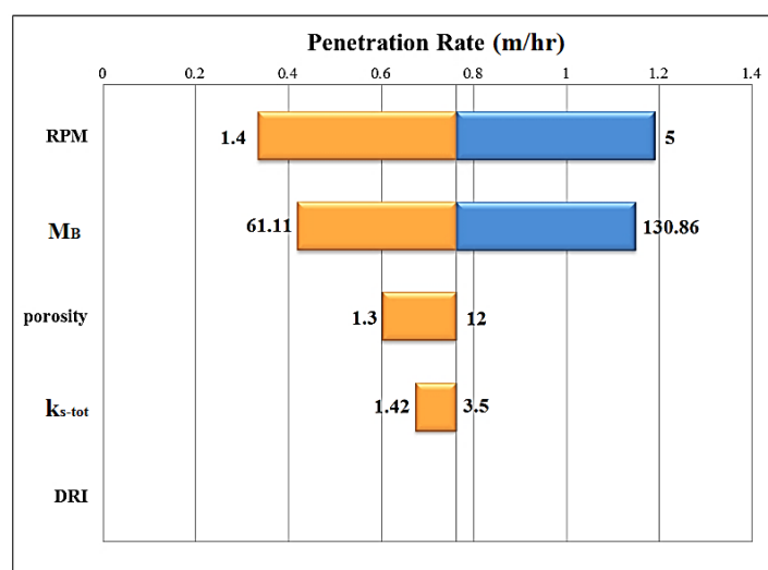
شکل ۶: نمودار گردباد تحلیل حساسیت مدل NTNU
