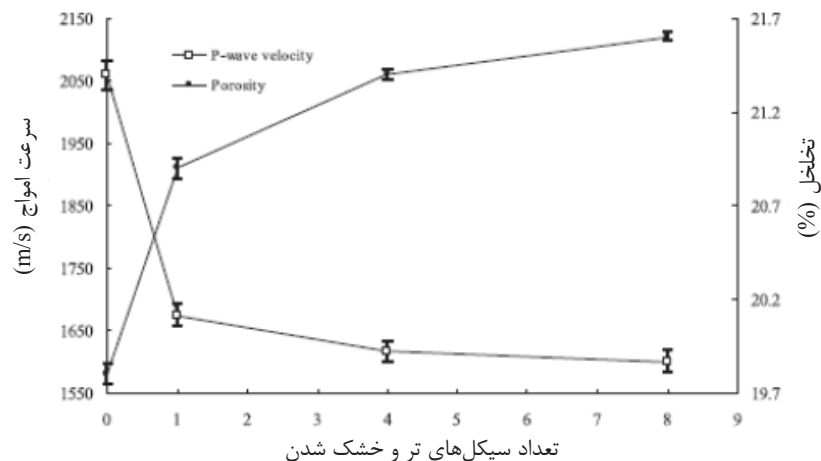
شکل ۳: تأثیر تعداد سیکل‌های تر و خشک شدن روی تخلخل و سرعت امواج طولی ماسه‌سنگ تری گورژ [۲]
