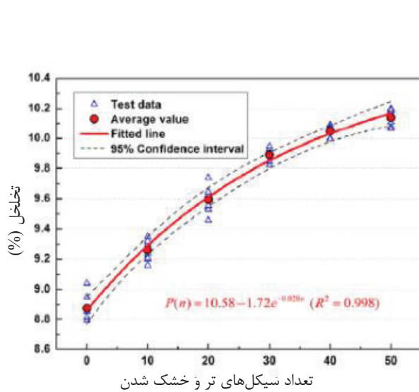
شکل ۲: رابطه بین تخلخل و تعداد سیکل‌های تر و خشک شدن [۳]
