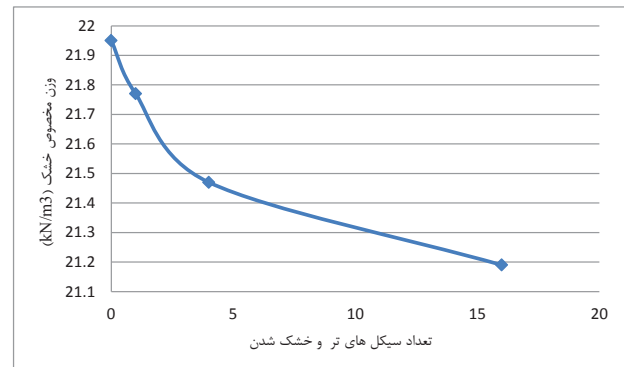
شکل ۸: روند تغییرات وزن مخصوص خشک با افزایش تعداد سیکل‌های تر و خشک شدن
